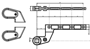
AC583 Braccio universale reversibile con forature
