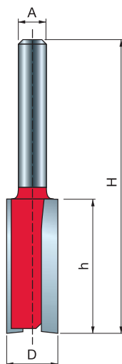
Tipo C Taglienti in HW saldobrasati
