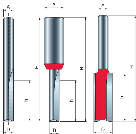
Tipo A Frese integrali in HW
