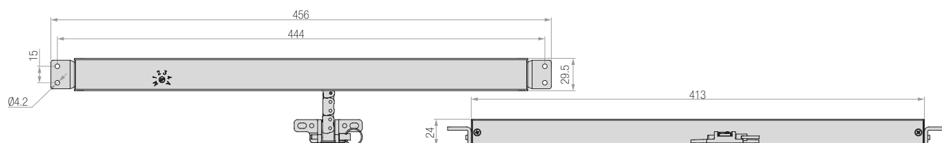
Vasistas interno Internal Bottom hung
