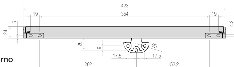
Vasistas esterno External Bottom hung
